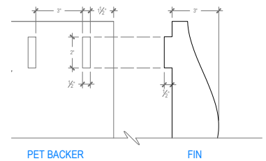
TYP Dimensions
