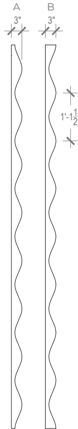
Fin Profiles
